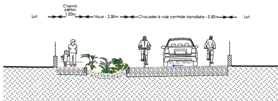
Coupe type emprise voirie 1 Sans échelle
