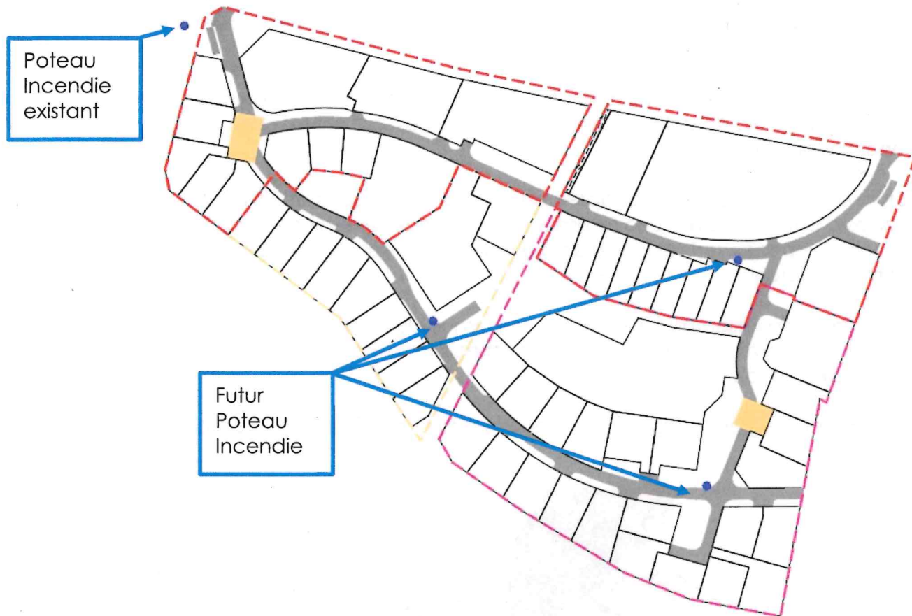
Plan de la défense incendie du projet
